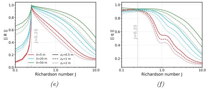
FIGURE 3.8 – Coefficient de réflexion à la surface : (a), (c), (e) à la sortie de la couche interne, (b), (d), (f) dans la région extérieure dans le cas cisaillement variable hydrostatique pour différentes valeurs de sld .
