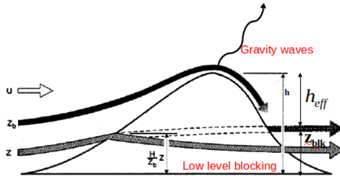
FIGURE 6.1 – Schéma explicatif de la paramétrisation SSO
