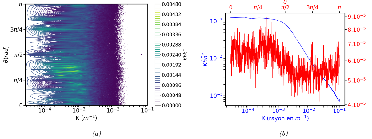
FIGURE 6.7 – Spectre de l'orographie : a) double transformée de Fourier tracée en fonction des coordonnées polaires, b) intégration en \theta (en rouge) et en K (en bleu)
