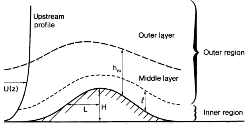
FIGURE 2.7 – Régions de l'écoulement (modifié depuis Carruthers and Hunt (1990))
